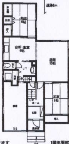
1階平面図
